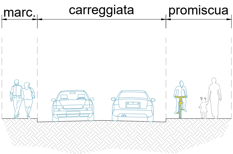
SEZIONE TIPO PISTA CICLABILE PROMISCUA SU MARCIAPIEDE*
