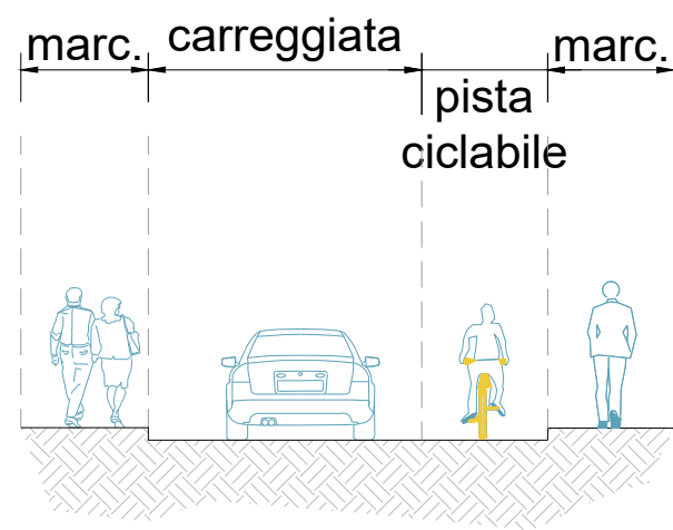
SEZIONE TIPO PISTA CICLABILE PROMISCUA SU STRADA*
