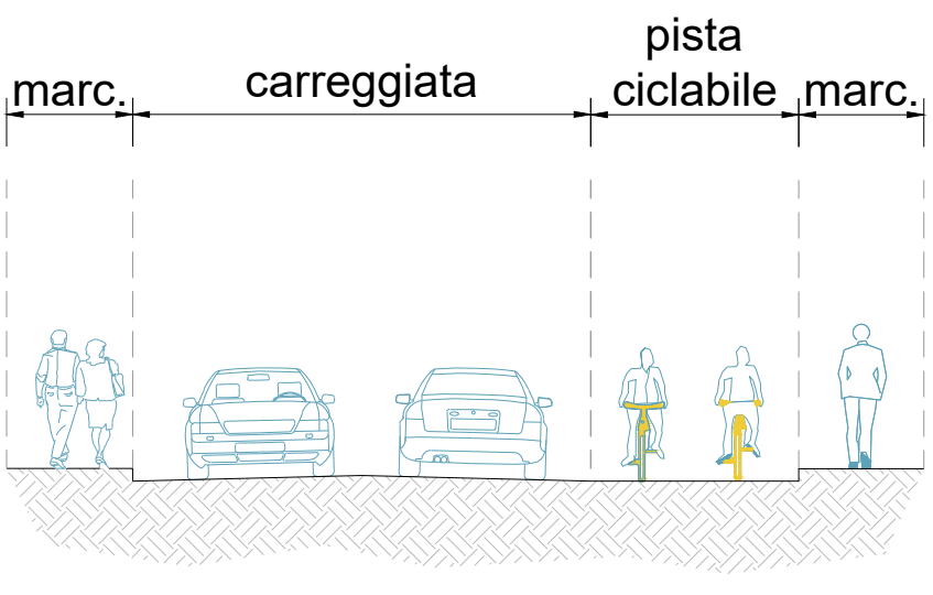
SEZIONE TIPO PISTA CICLABILE IN CORSIA RISERVATA*
