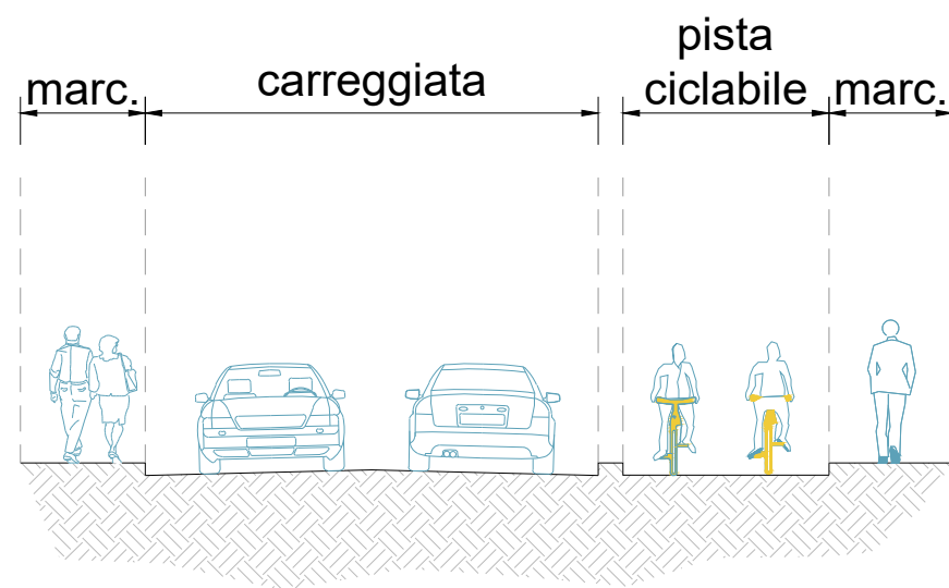
SEZIONE TIPO PISTA CICLABILE IN SEDE PROPRIA*
